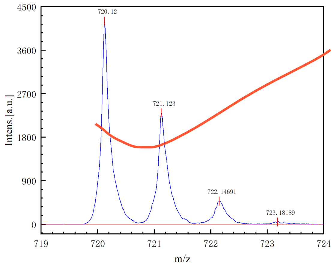
图 2 C 60 的负离子模式激光解吸飞行时间质谱
